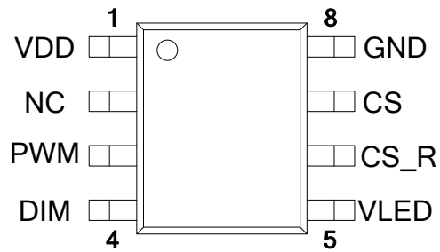
ESOP8
