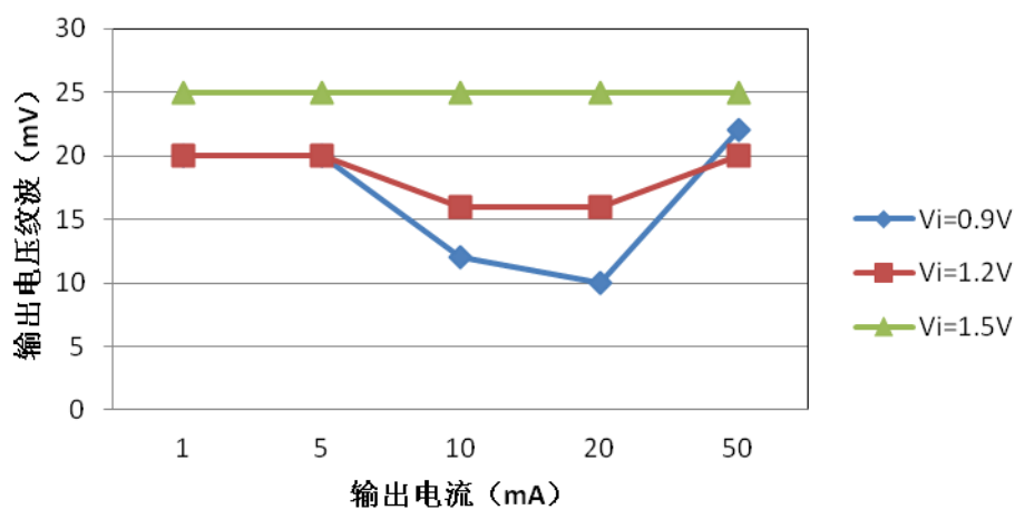
输出电压纹波与输出电流
