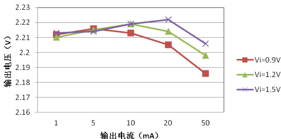
输出电压与输出电流
