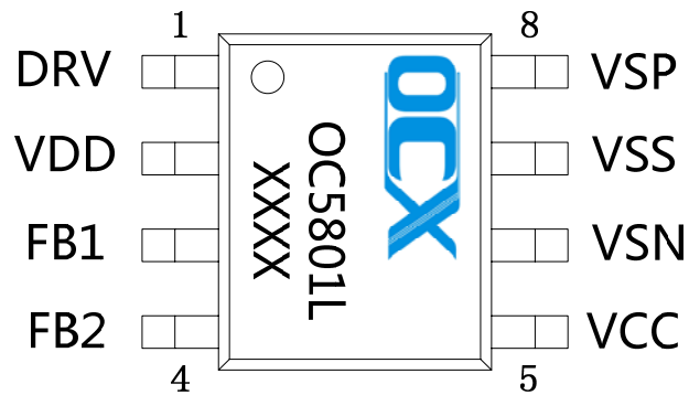
SOP8
