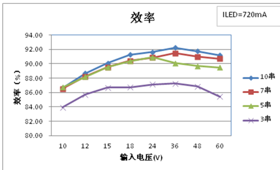
转换效率与输入电压&LED 串数量
